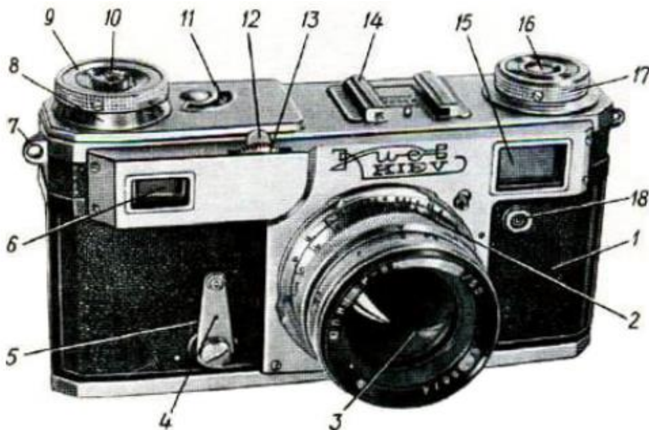
Рис. 2. Общий вид фотоаппарата
