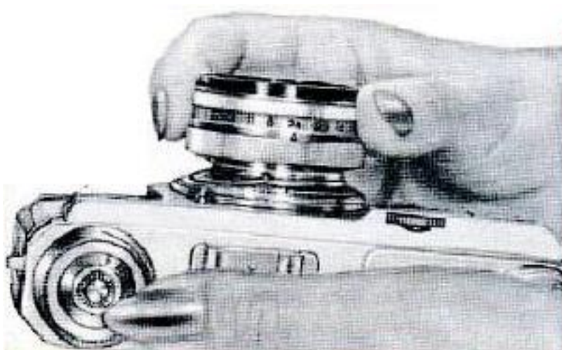
Рис. 15. Диафрагмирование объектива
