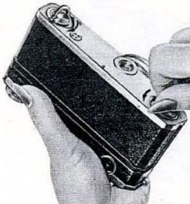
Рис. 6. Открывание замков на задней стенке
