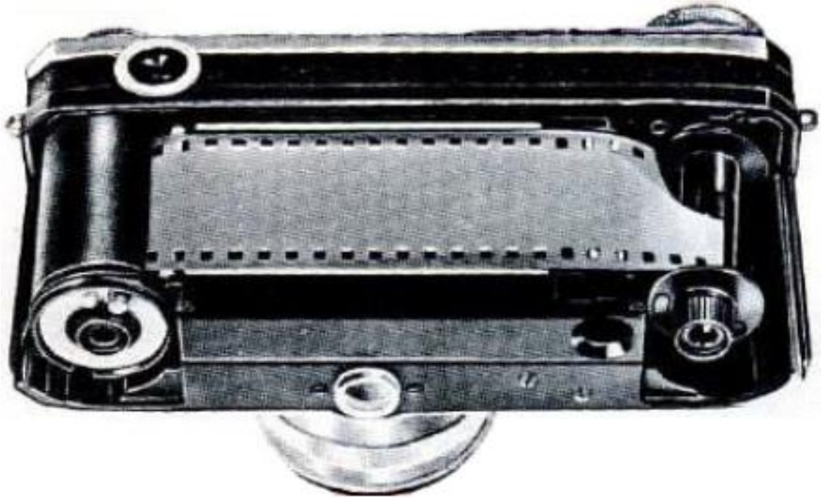
Рис. 11. Аппарат, заряженный кассетой и катушкой
