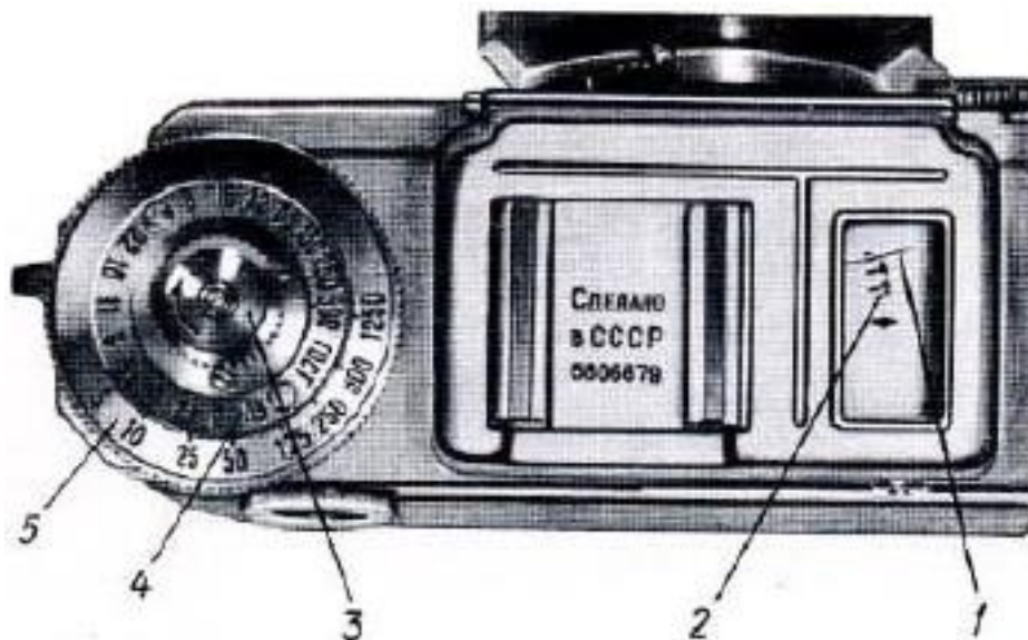
Рис. 24. Вид экспонометра сверху
