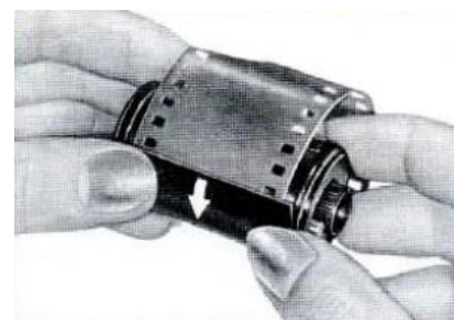
Рис. 10. Закрывание кассеты крышкой
