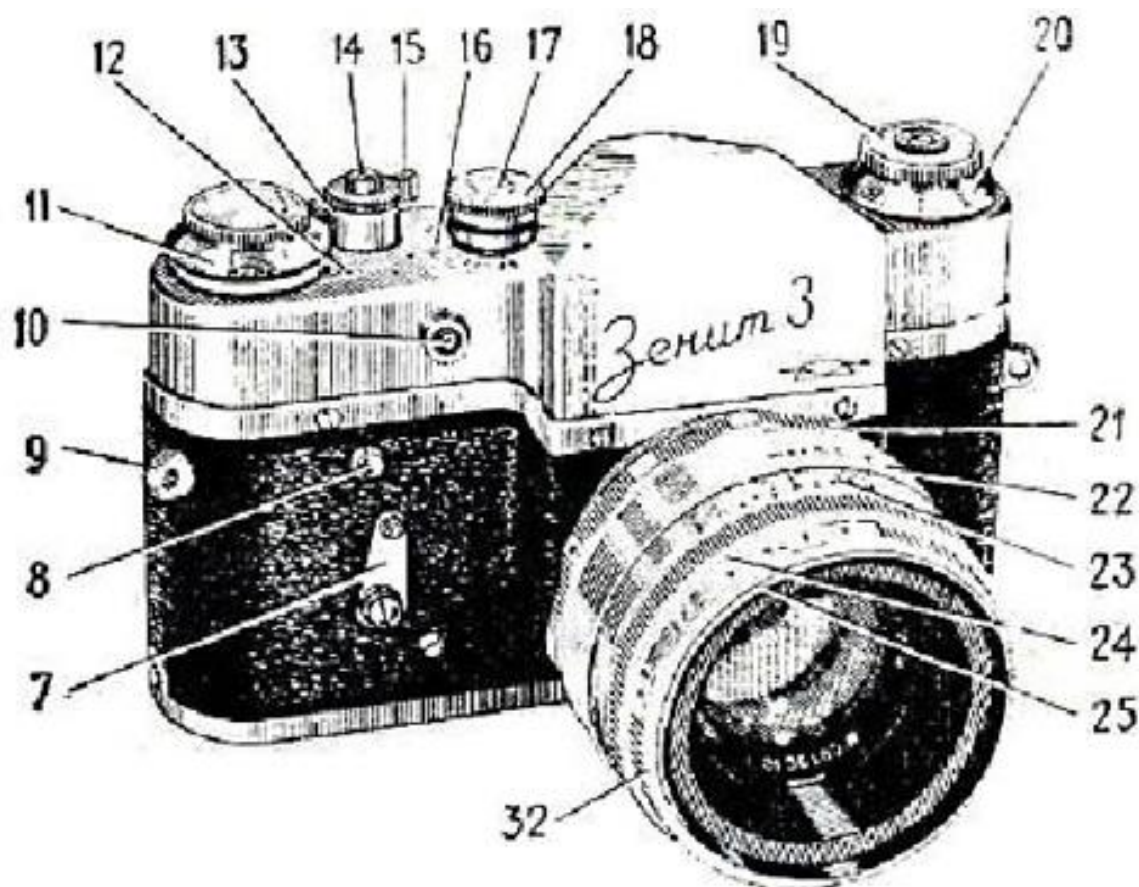
Рис. 2. Фотоаппарат «Зенит-3»
